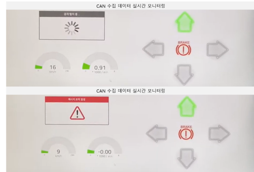
[그림 5] CAN 메시지 공격 탐지 화면
